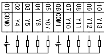
4.3寸一体机MM_20MR_6MT_430A_FX_F接线图
