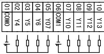
4.3寸一体机MM_20MR_6MT_430A_FX_A接线图 V2
